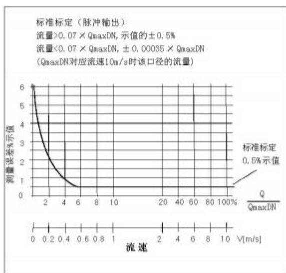
图 1 测量误差曲线
