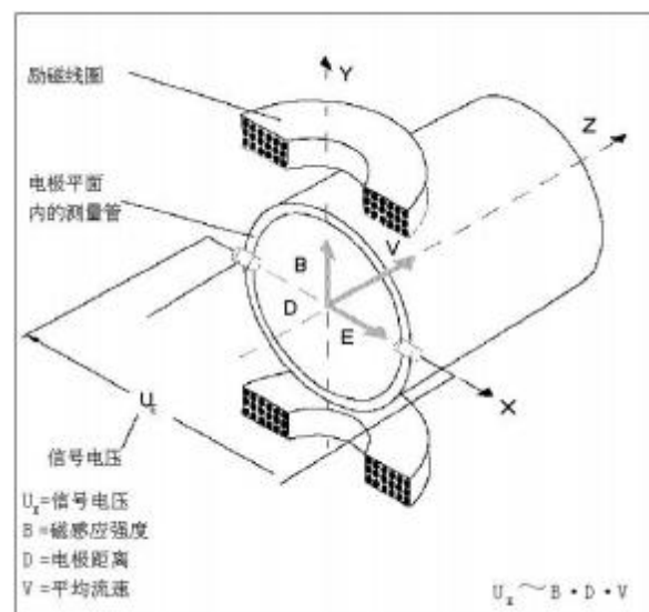
图 2 电磁流量计原理图
