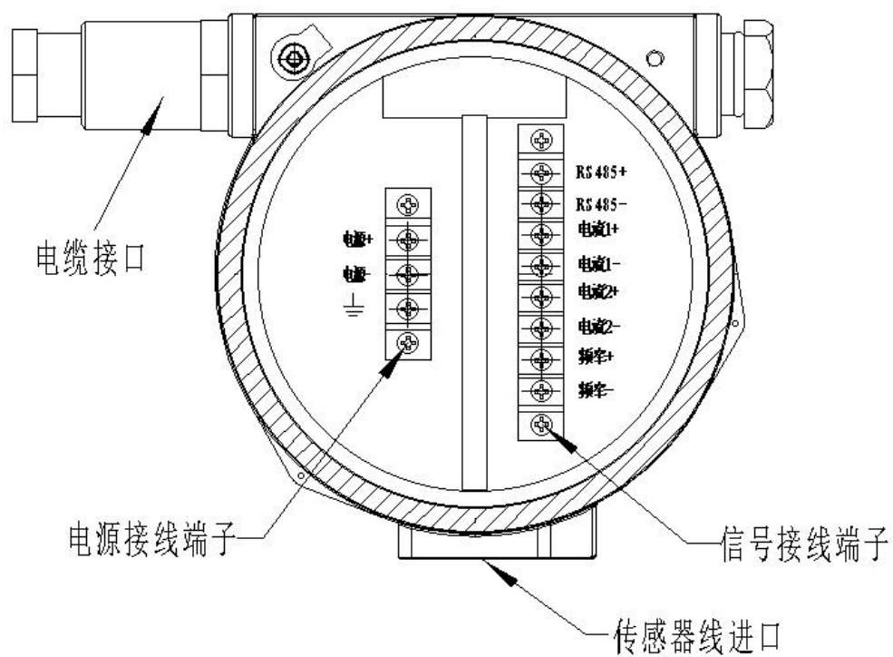
图 4 变送器接线图
