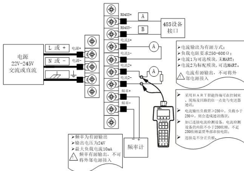
图 5 变送器接线关系图
