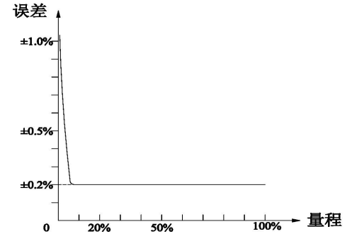
图 2 测量误差曲线
